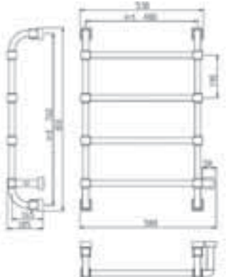
Scaldasalviette riscaldato in quadrati 25x25 tubo di ottone (acqua/elettrico). Fixed modular heated towel rail in squared brass tube 25x25 (combi water/electric). Настенный полотенцесушитель, латунь, трубка 25x25 (водяной / электрический).
